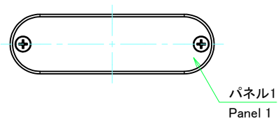
A-A (1:1.5)
